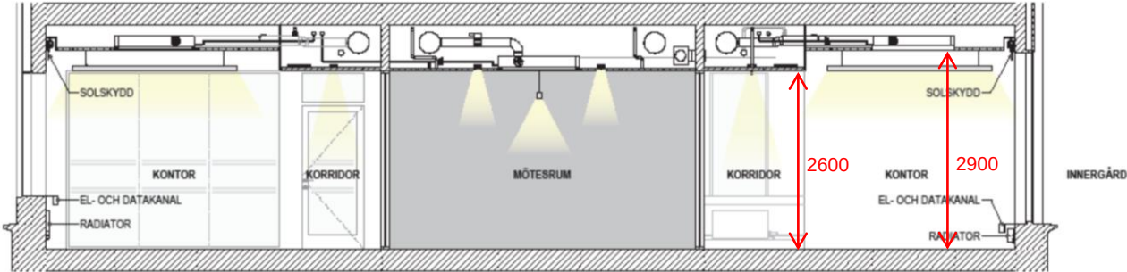
Principsektion
