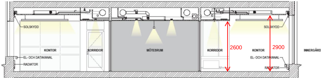
Principsektion
